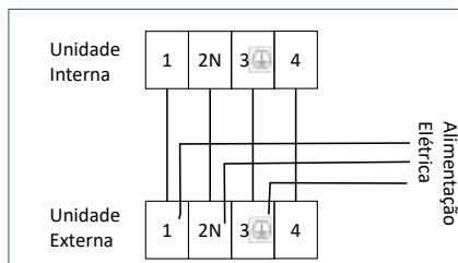
Diagrama de conexões para 30K e 36k
