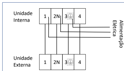
Diagrama de conexões para 9K, 12K, 18K e 24K
